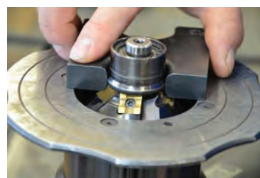
Radius edge milling depth setting tool
